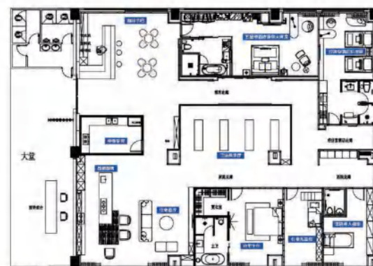
泉州工业化装修展示厅-平面布置图
